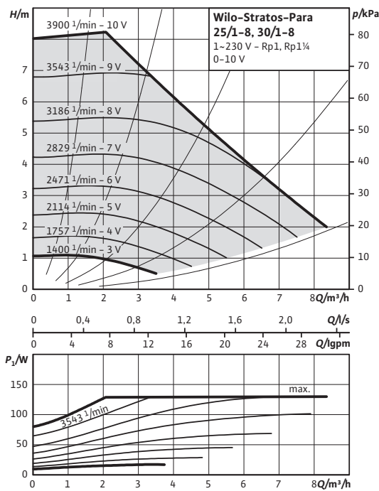
Wilo-Stratos PARA 25/1-8, 30/1-8
