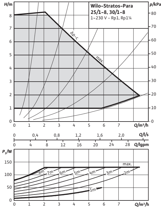
Wilo-Stratos PARA 25/1-8, 30/1-8
